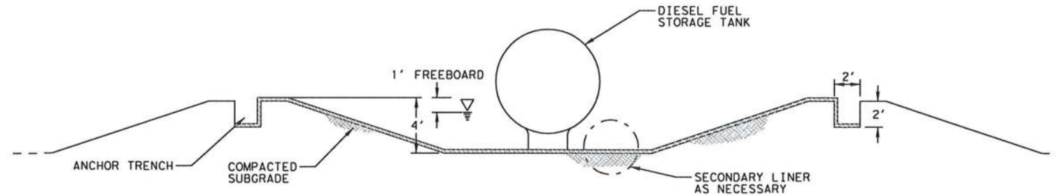
TYPICAL DIESEL FUEL TANK N. T. S.
