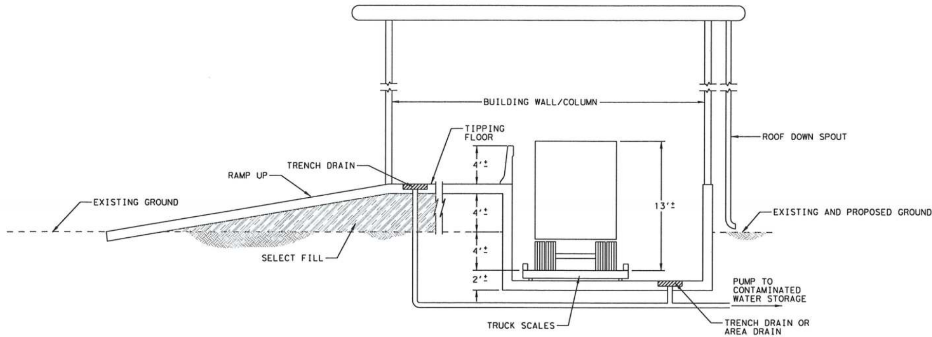
SCHEMATIC CROSS SECTION N. T. S.
